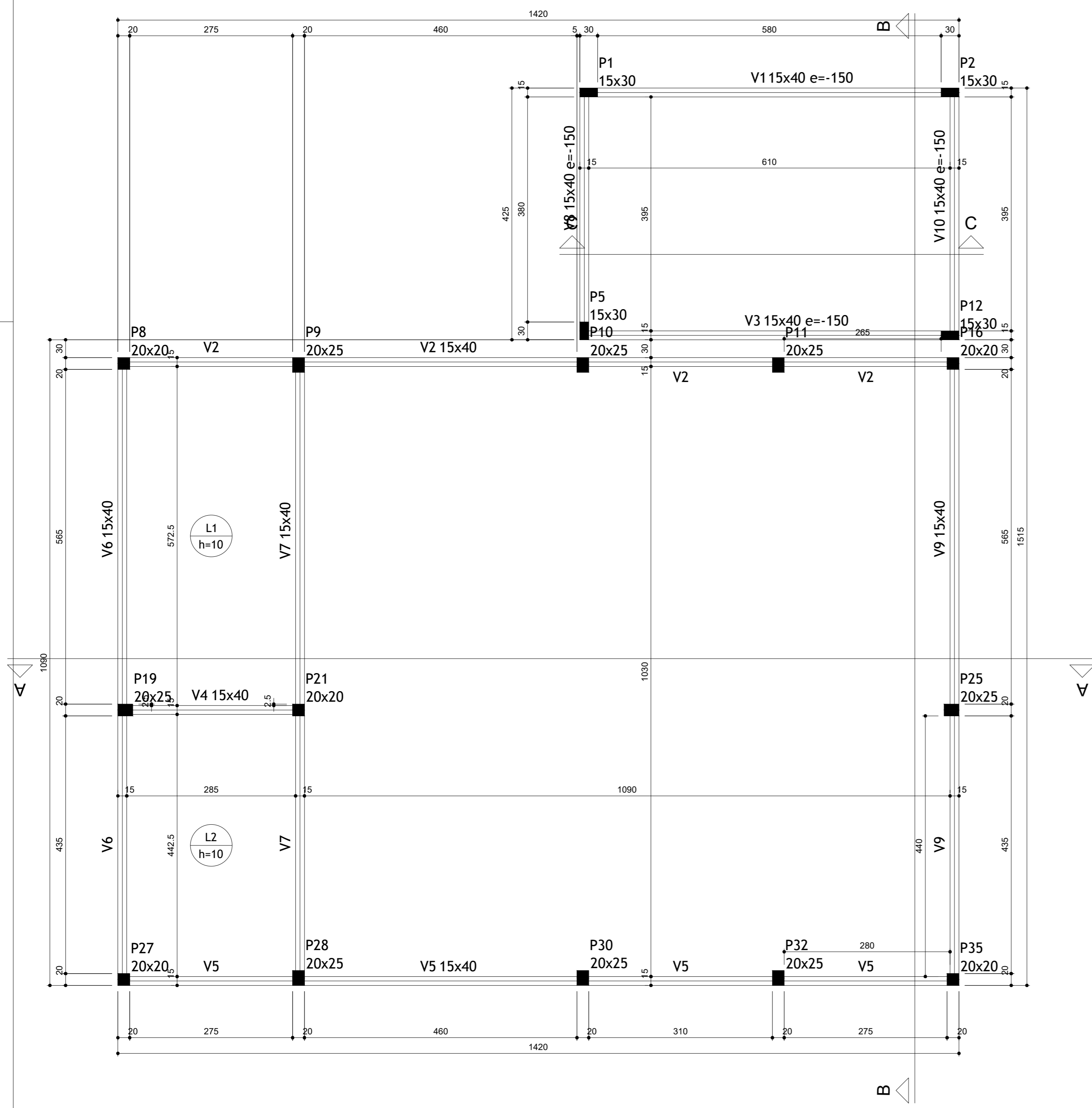
Forma do pavimento Cobertura (Nível 860) escala 1:50
