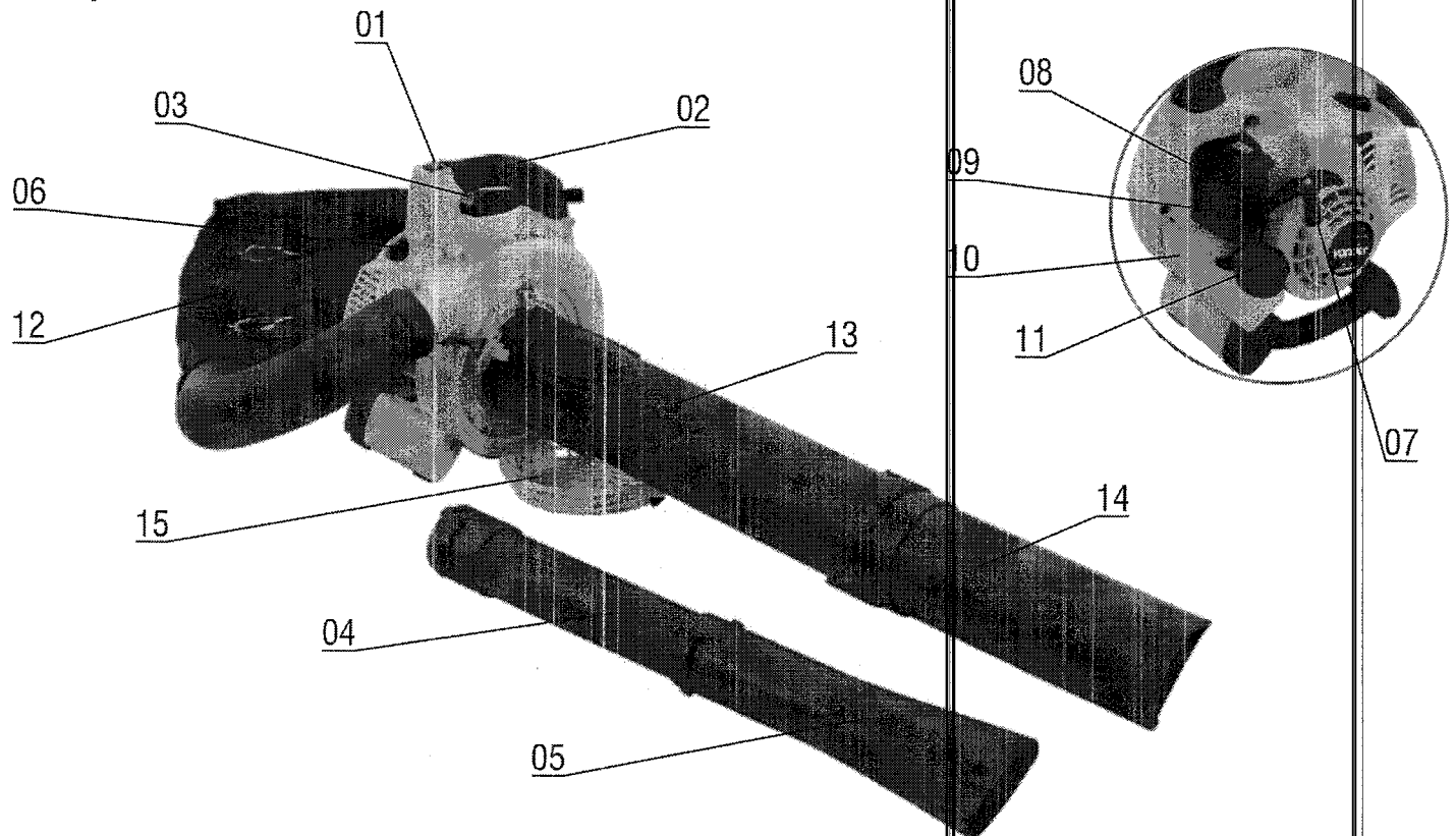
Fig. 2 – Componentes
