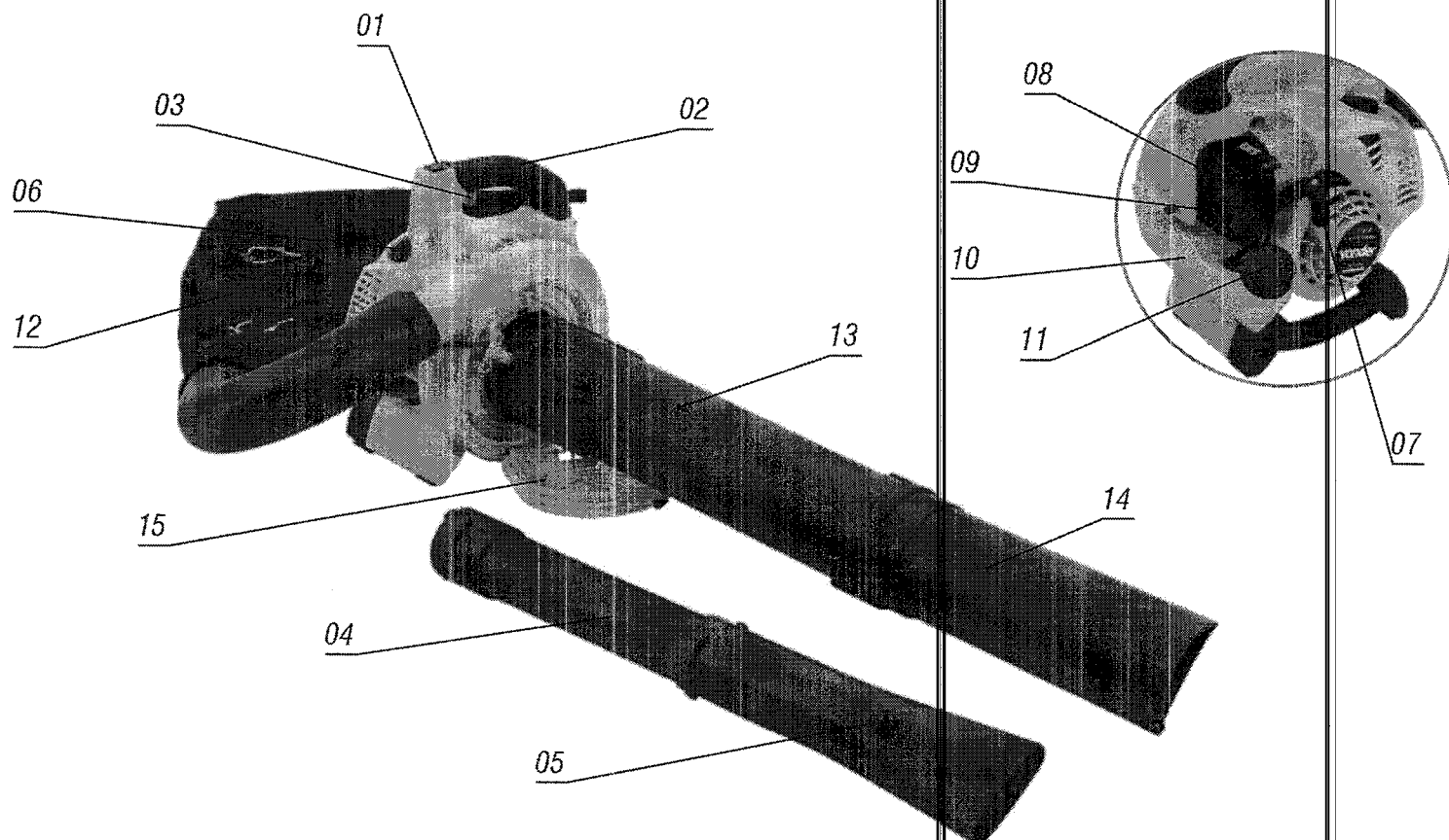
Fig. 2 – Componentes
