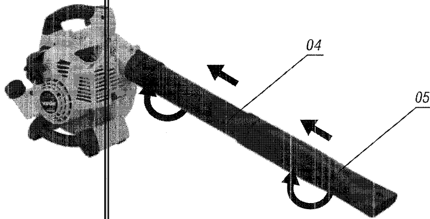
Fig. 3 – Montaje del tubo del soplador
