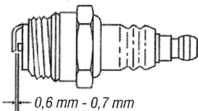
Fig. 10 – Huelga de la bujía
