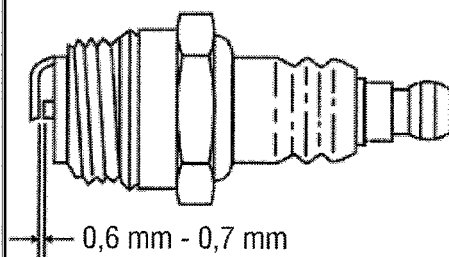
Fig. 10 – Folga da vela
