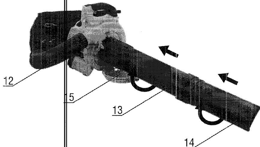
Fig. 4 – Montagem dos tubos para o aspirador
