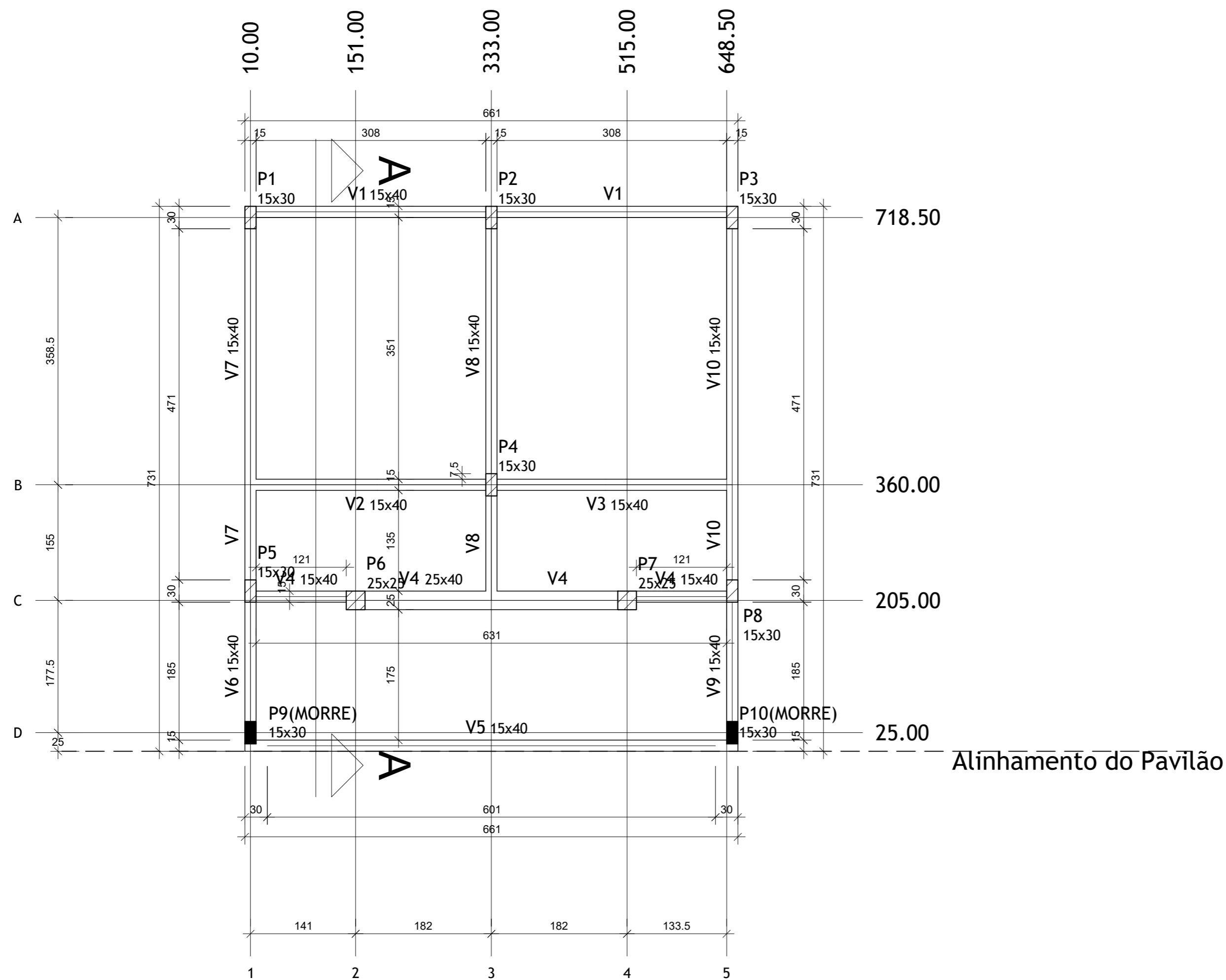
Forma do pavimento Térreo (Nível 0) escala 1:100
