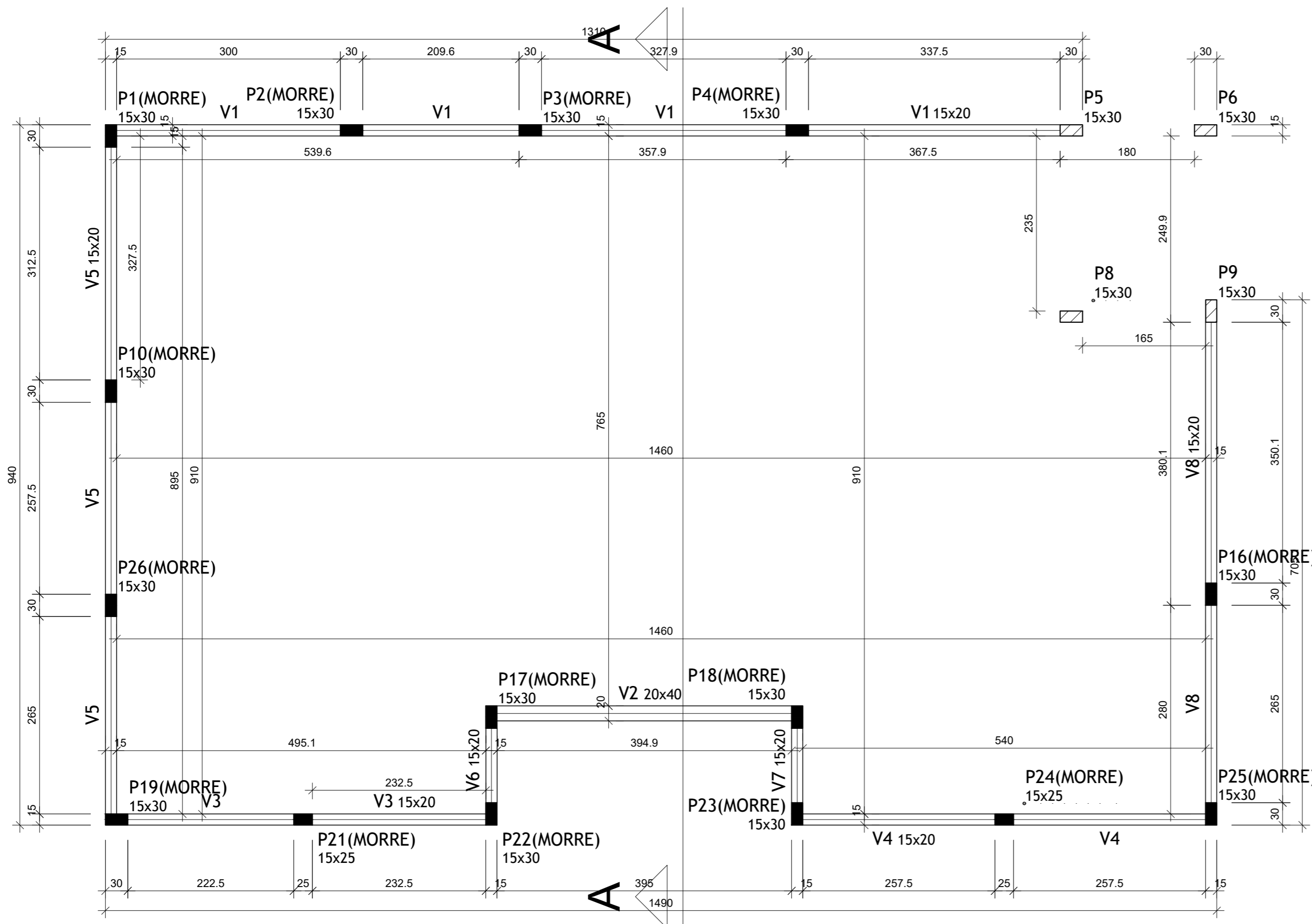
Forma do pavimento Platibanda (Nível 420) escala 1:50
