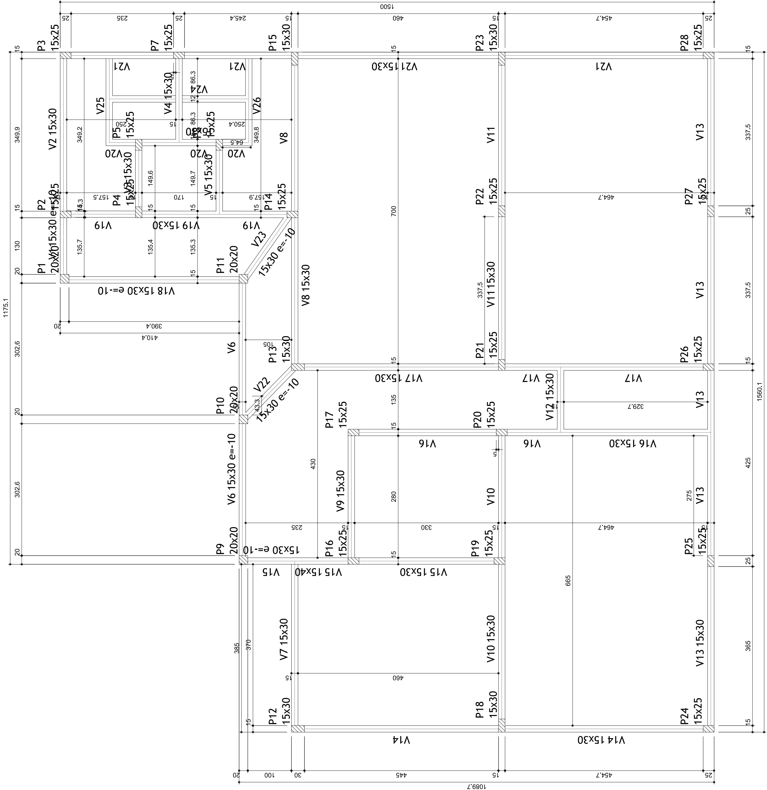
Forma do pavimento Baldrame (Nível 0) escala 1:50
