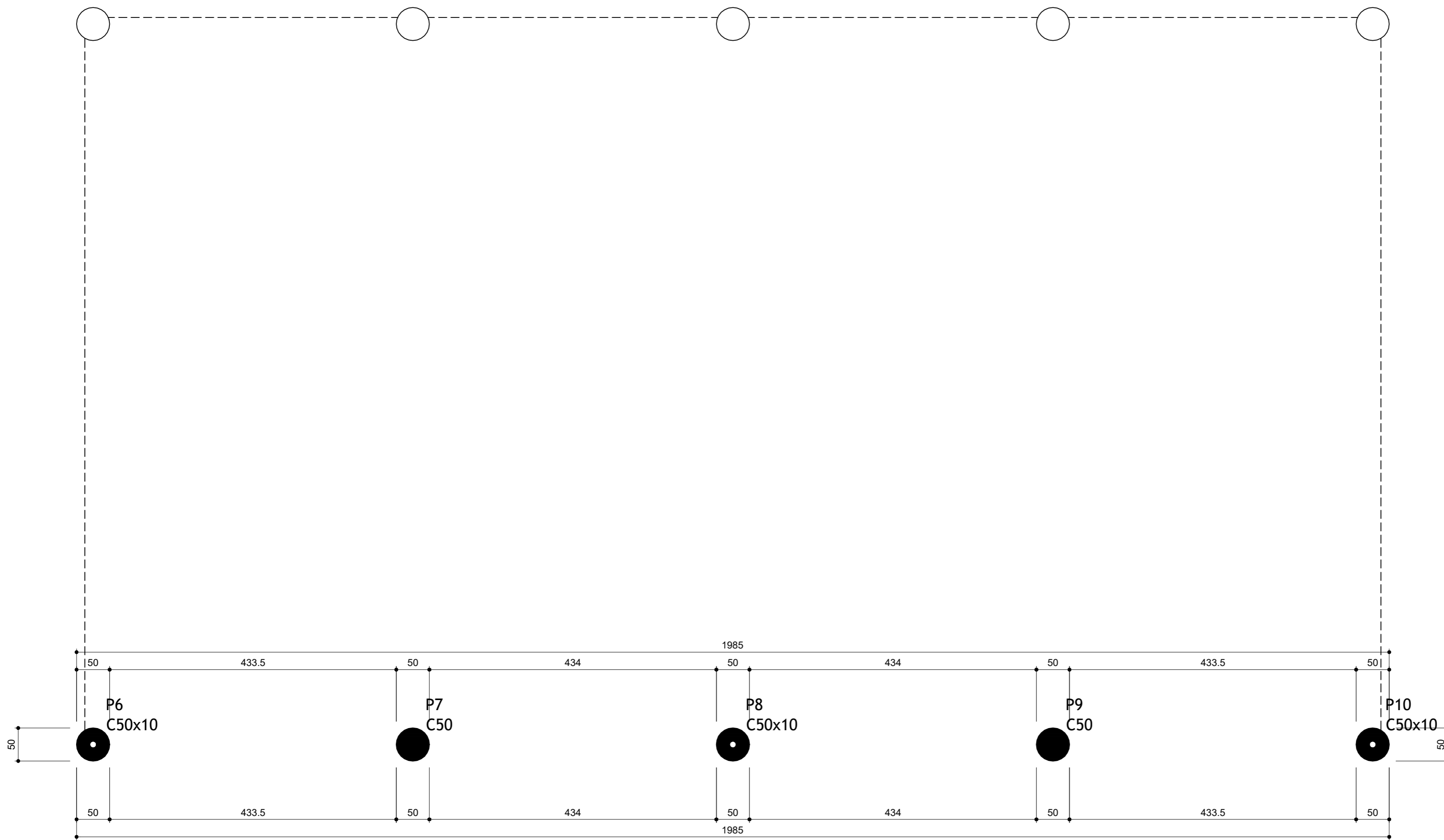
Forma do pavimento Tirante (Nível 850) escala 1:50
